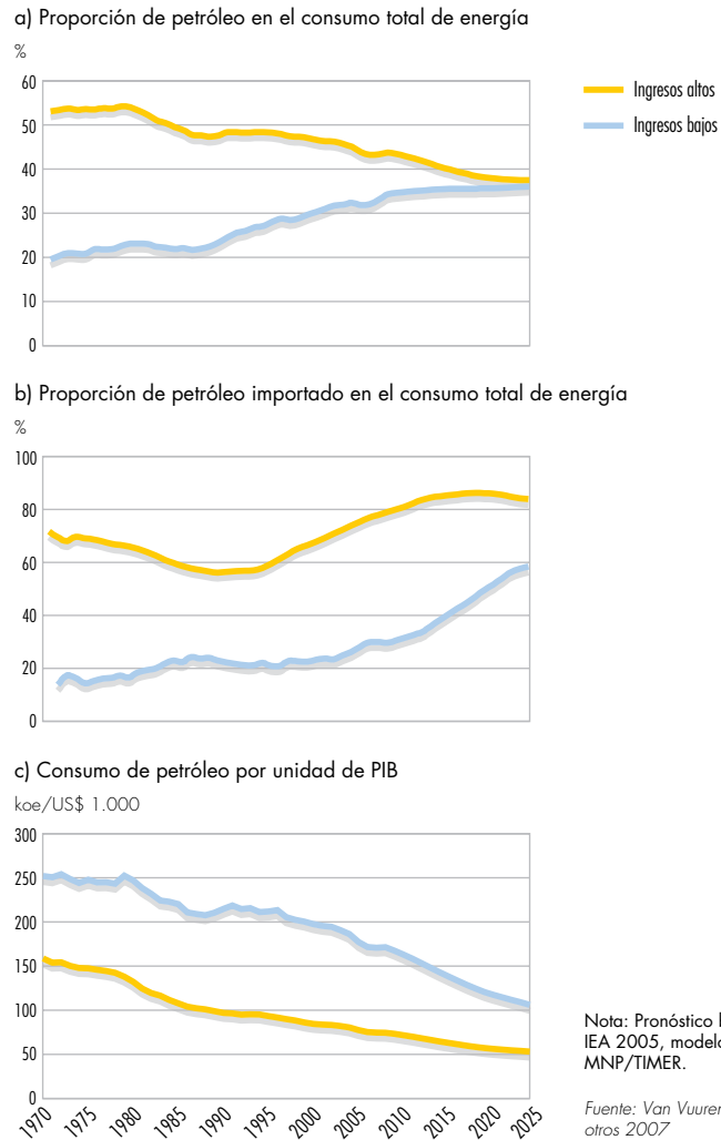
Figura 7.20 Tendencias y proyecciones en la seguridad de petróleo para regiones importadoras de energía de ingresos altos y bajos
