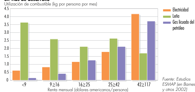
Figura 5.6 Relación entre renta y utilización de energía en zonas urbanas de 12 países en vías de desarrollo
